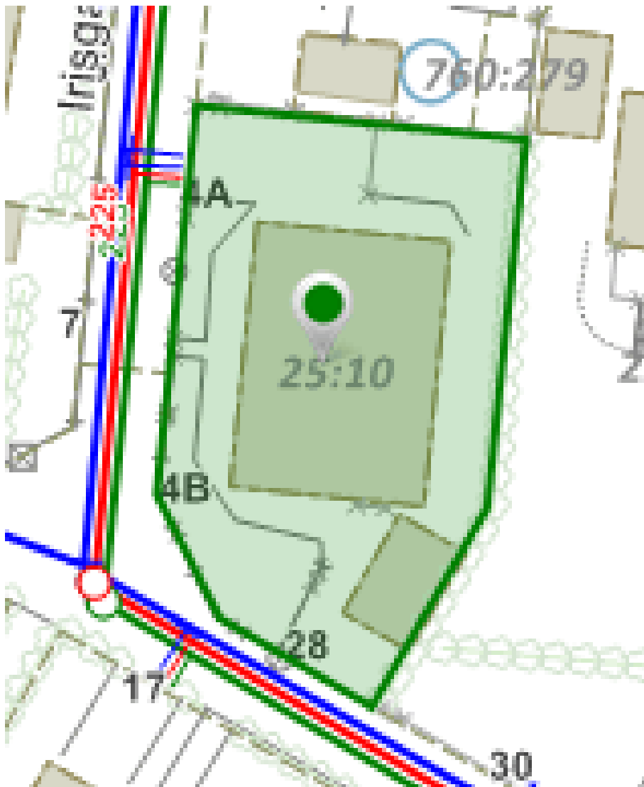
Figur 3: Ledningskarta, Kretslopp och vatten (Kov)
